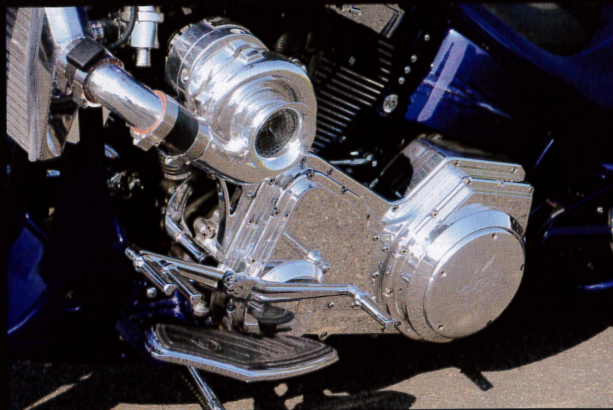
動力にプライマリーを利用するプロチャージャー。メーカーでは馬力とトルクが50~70パーセント向上すると謳っている
